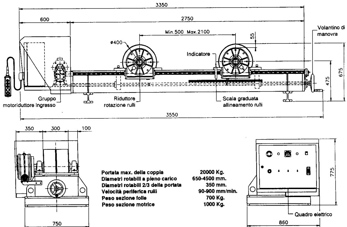
POSIZIONATORE A RULLI mod.PR200
